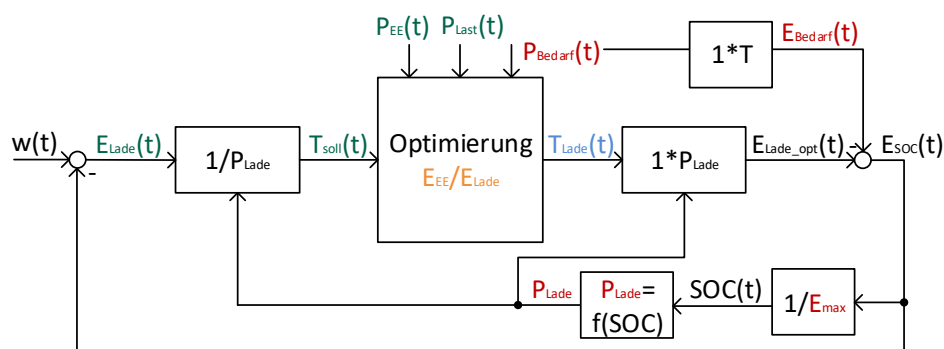
Abbildung 3: Regelkreis zur Beschreibung einer Laderegelung eines Elektrofahrzeuges aus energie-technischer Sicht
